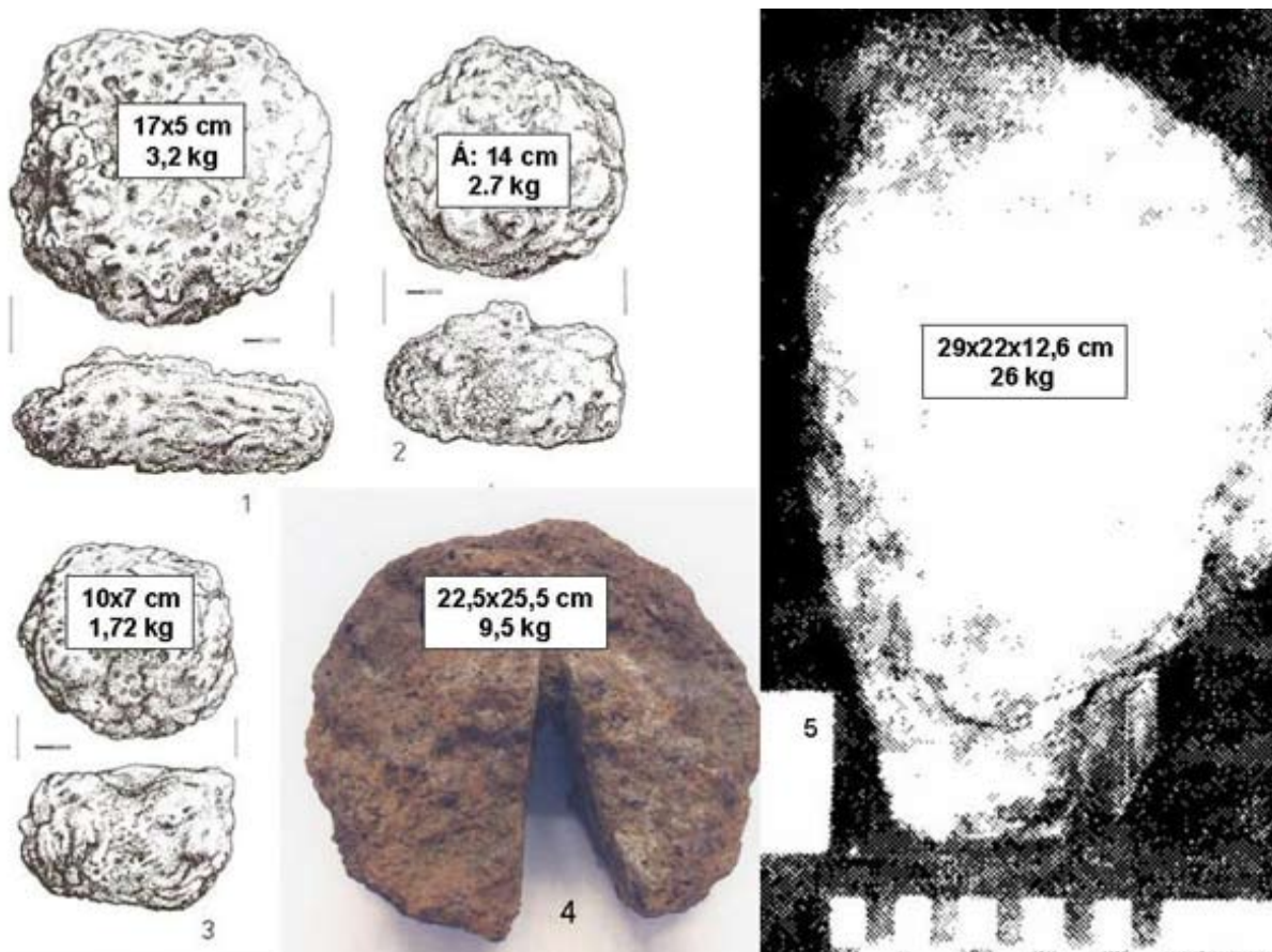
1. ábra. Somogy megyei vasbucacaletek. 1–3. Somogyfajsz-Ívató tó, 10. század végi vasolvasztó műhely (GÖMÖRI 2000, 155.), Óskohó Múzeum, Somogyfajsz; 4. Lábod-Petesmalom, 8–9. század (KÖLTŐ – FEHER 2016.) Rippl-Rónai Múzeum, Kaposvár; 5: Szalacska, (HEGEDŰS 1961, XVI. tábla, 2, mint középkori félbuca; SÁGI 1979; ROZSNOKI 1979, 1d. ábra, mint késő róma, 4–5. századi félbuca. Központi Kohászati Múzeum, Miskolc-Diósgyőr
