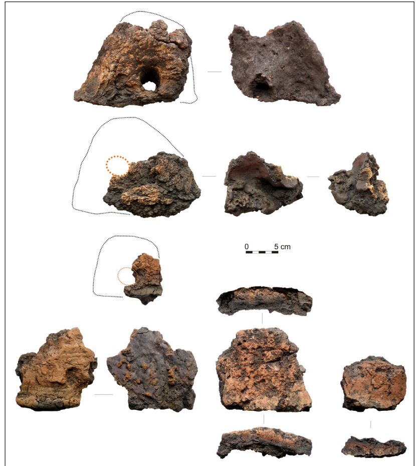
7. kép: Kürtő alakú, felszínre épített vasolvasztó kohó darabjai Csíksomlyó-árvaház lelőhelyről
