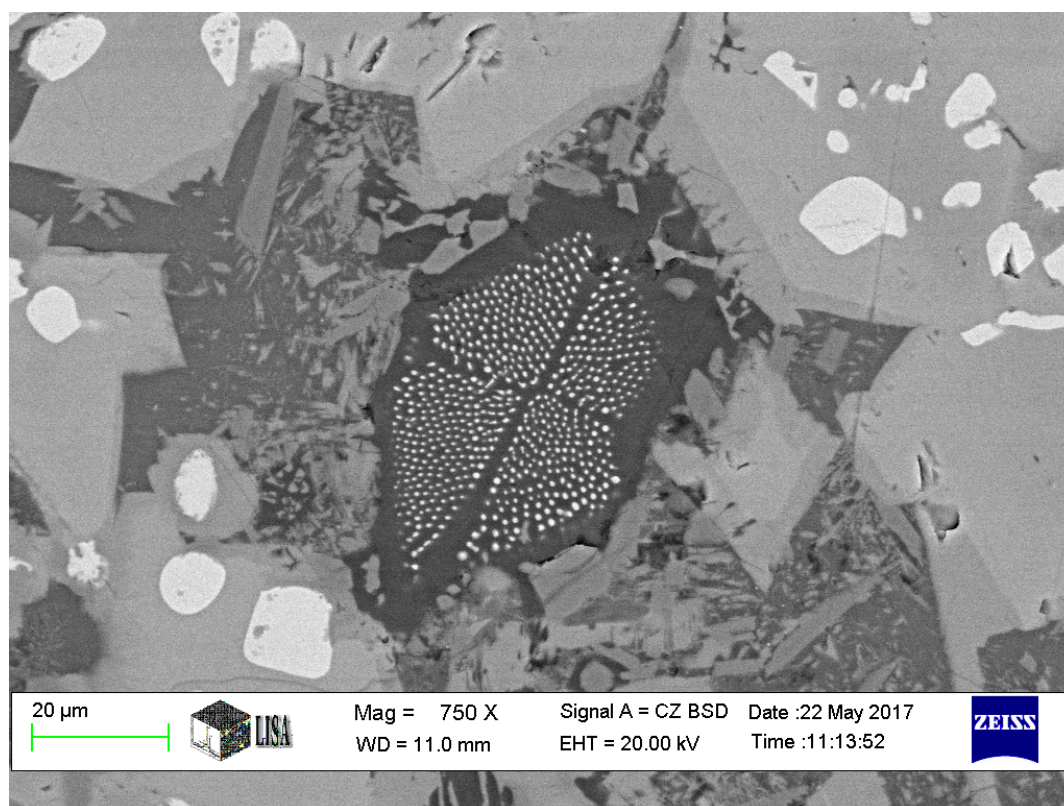
6. ábra: Kálium-dús közegben pontszerű mintában eloszlott wüstit, fayalitos részekkel (szürke) és vas-oxid szemcsékkal (fehér – O: 12,32 tömeg%, Fe: 82,65 tömeg%) körülvéve.
